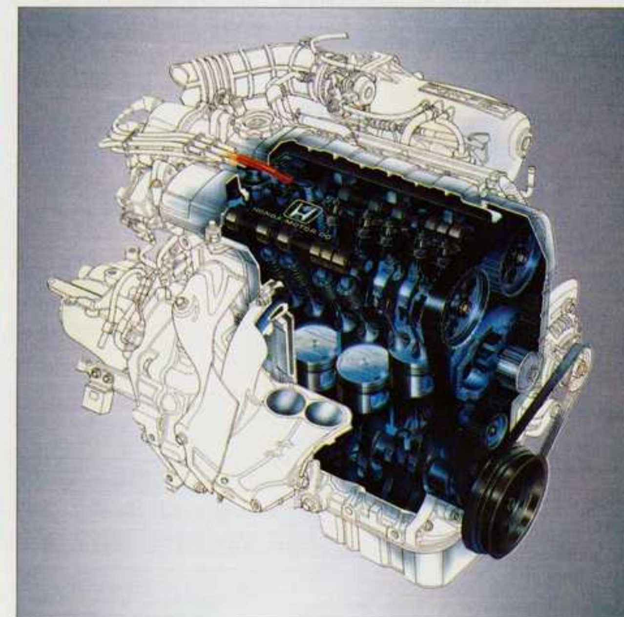
Moteur 16 soupapes 1.6i - 16 DOHC 122 CH*. Injection électronique PGM-FI
