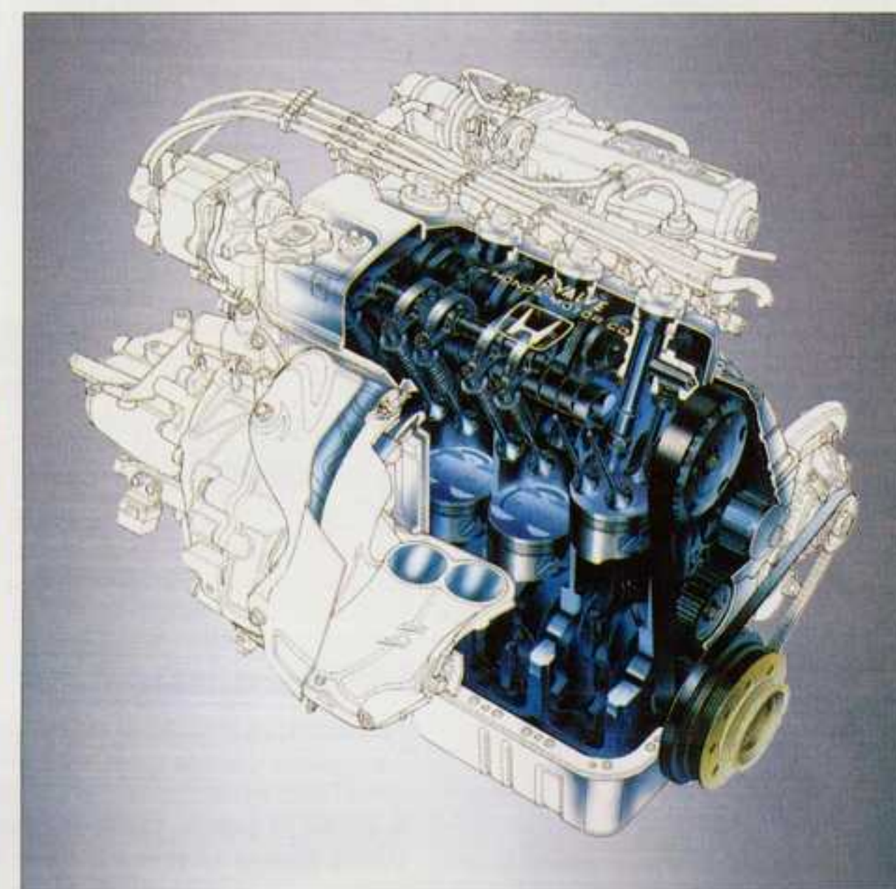
Moteur 16 soupapes SOHC, 111 CH* Injection électronique PGM-FI
