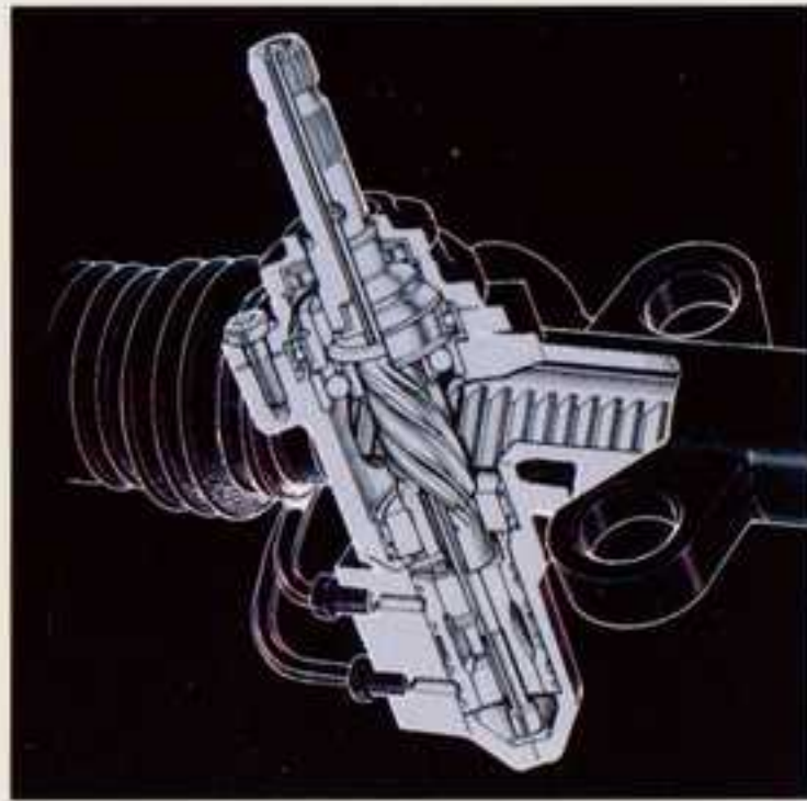
Direction assistée pour une conduite souple et sûre
