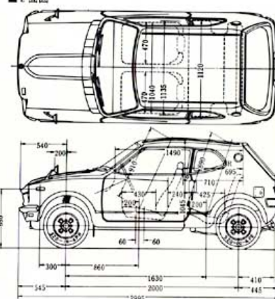
■2面図
