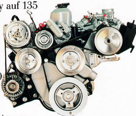
Der 4L Sechszylindermotor: 135 kW (184 PS) bei 4750 min -1 , maximales Drehmoment von 290 Nm bei 3950 min -1 .
