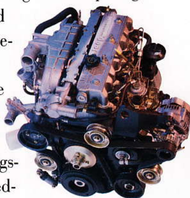
Der neue 2,5L Turbodiesel-Motor leistet 85 kW (116 PS) bei 4000 min -1 und ein maximales Drehmoment von 280 Nm bei 2000 min -1 .
