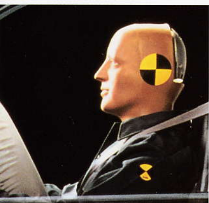
Der Lenkrad-Airbag entfaltet sich innert 20 Millisekunden. Er wird im Falle einer Frontalkollision bei über 19 km/h automatisch aktiviert.
