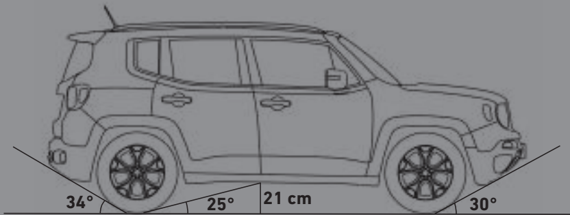
Угол въезда — 30°/ Угол продольной проходимости— 25°/ Угол съезда — 34°
