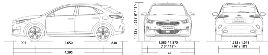
Abmessungen (mm)
