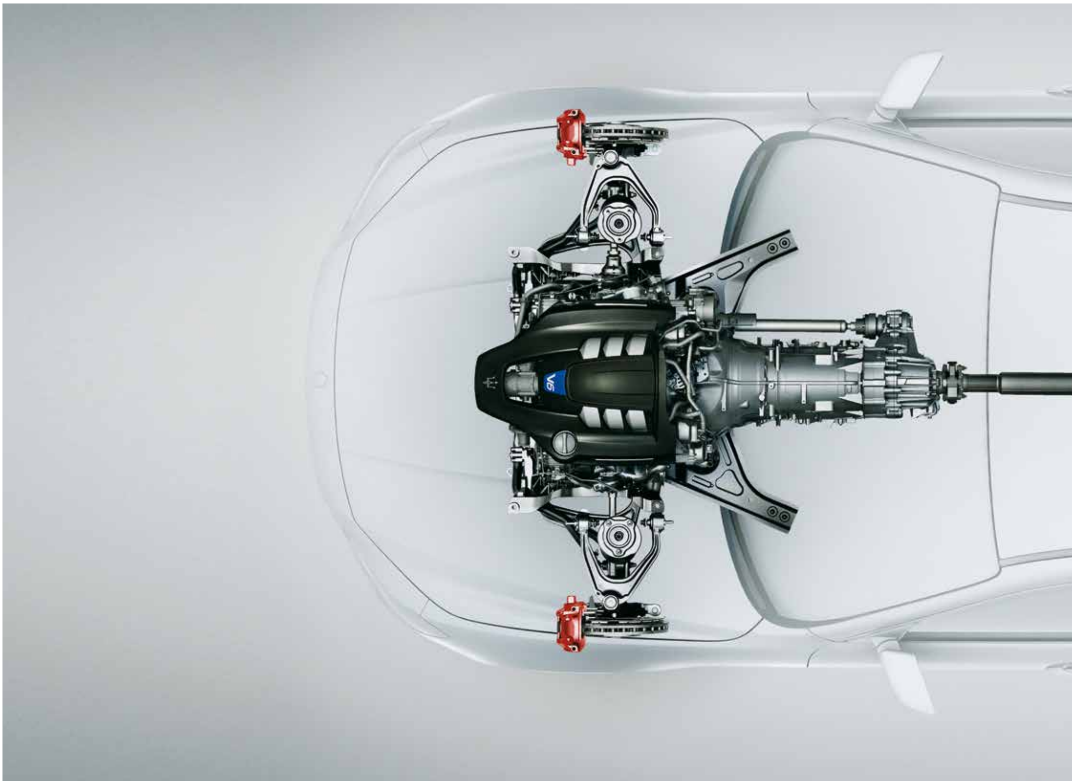
GHIBLI S Q4轿车采用全轮驱动系统，按需分配牵引力
