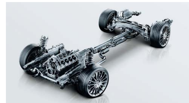
AMGスポーツサスペンション
