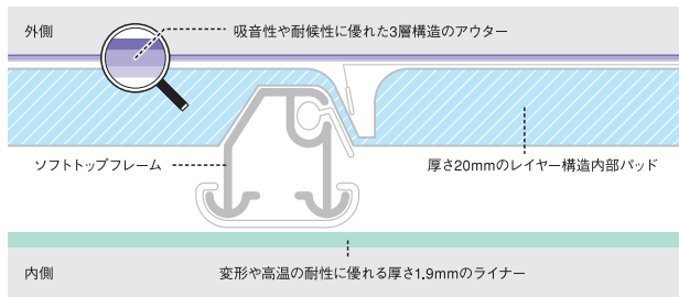
新素材を多用したアコースティックソフトトップの構造
