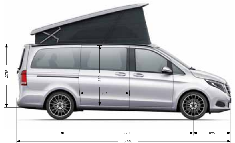
Vista lateral con techo elevable abierto
