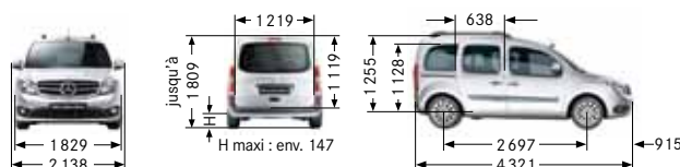
Citan Tourer long avec empattement de 2 697 mm
