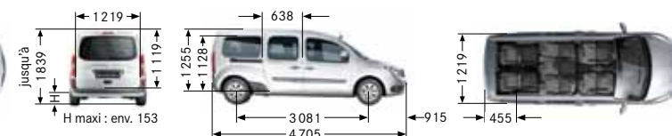
Citan Tourer extra long avec empattement de 3 081 mm
