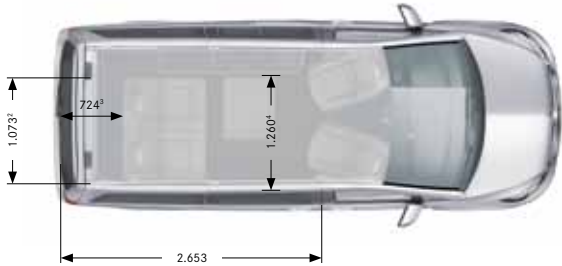
Banco en posición de asiento
