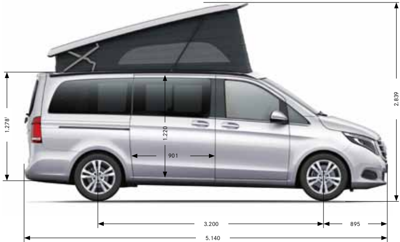
Lateral con techo elevable abierto
