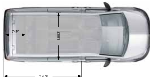
Banco en posición de asiento
