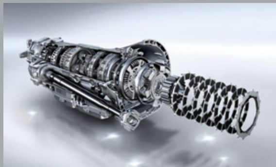
AMG SPEEDSHIFT MCT 7速运动型变速箱
