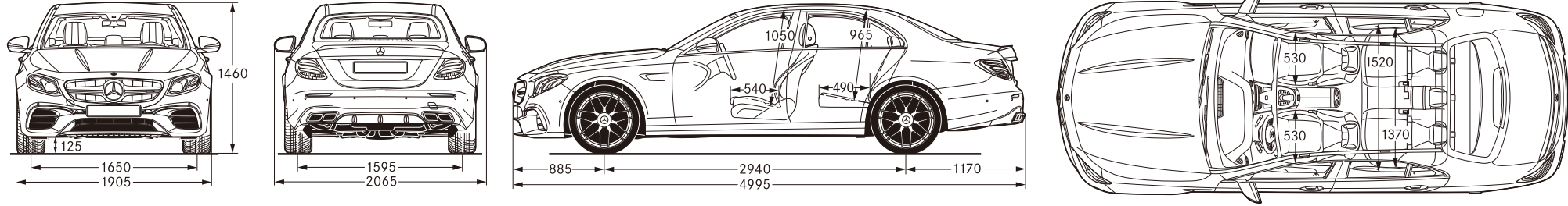
単位：mm
