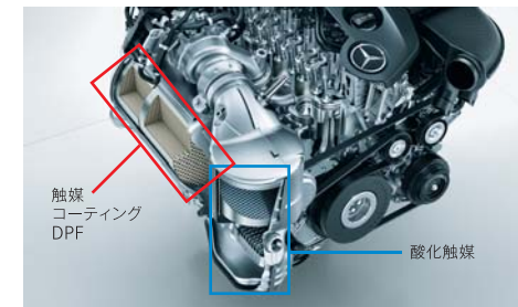
排出ガス浄化システム
