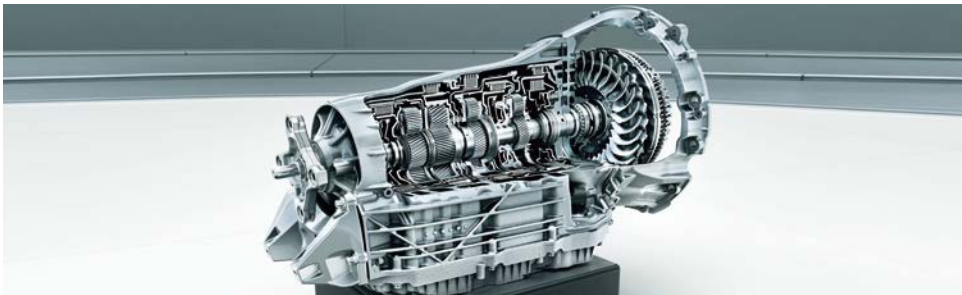
快適性、効率性、俊敏性を備えた 電子制御9速A/T、9G-TRONIC
