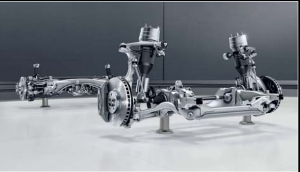
AMGスポーツサスペンション(AIR BODY CONTROL)
