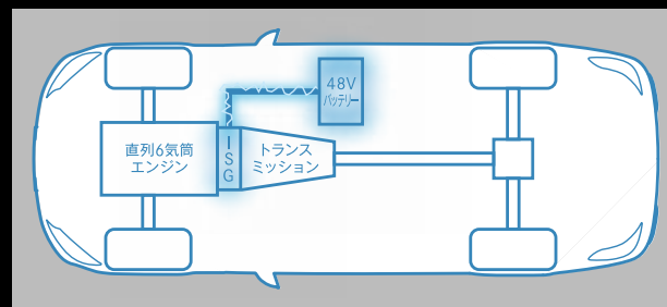
ISG(Integrated Starter Generator)イメージ
