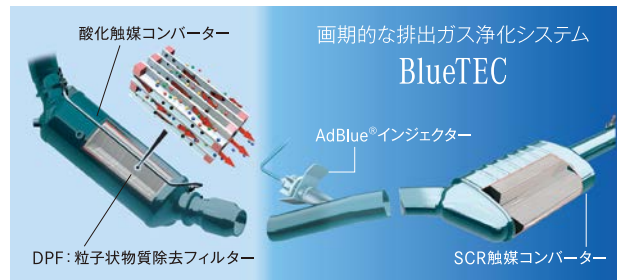
排出ガス浄化システムBlueTEC
