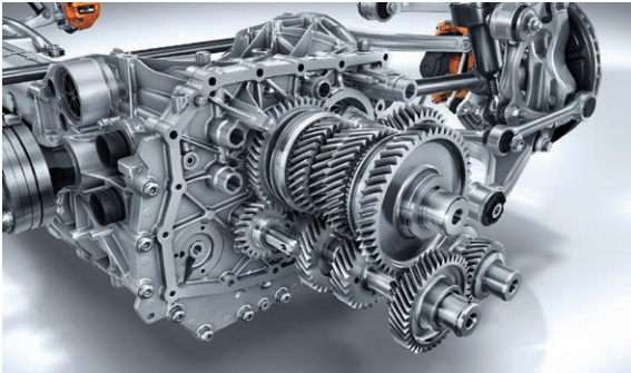
AMG SPEEDSHIFT DCT 7速运动型双离合器变速箱
