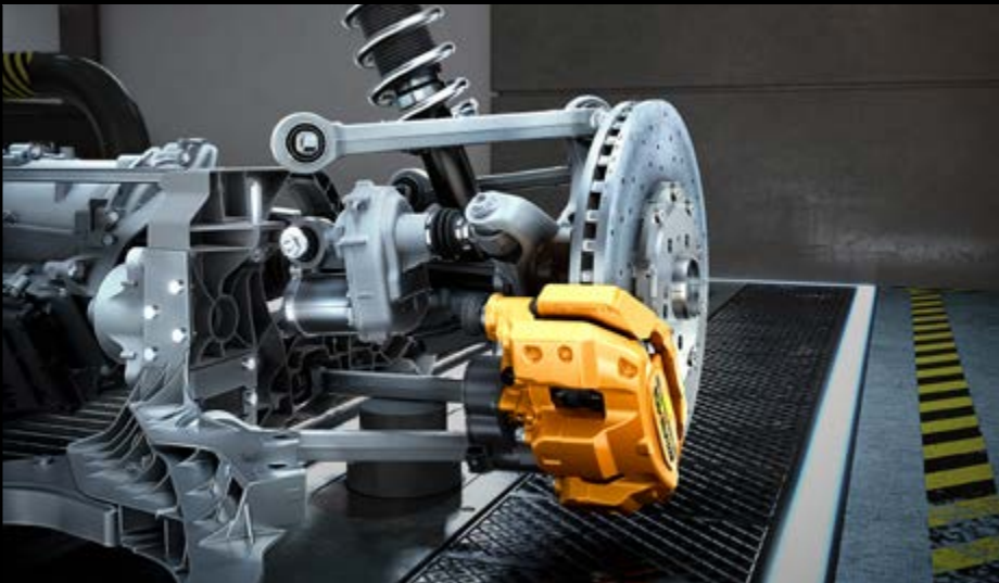
AMG Hinterachslenkung (201)
