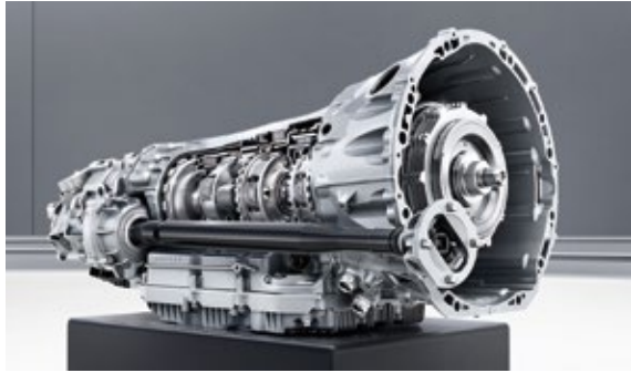
AMG SPEEDSHIFT TCT 9速自动变速箱
