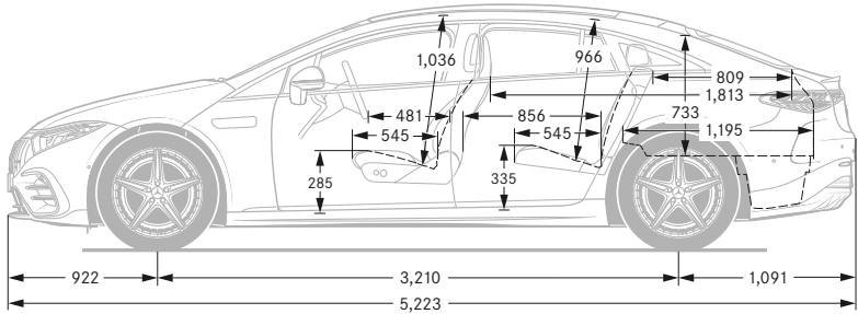
Mercedes-AMG EQS 53
