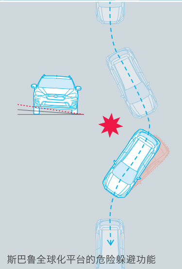
斯巴鲁全球化平台的危险躲避功能
