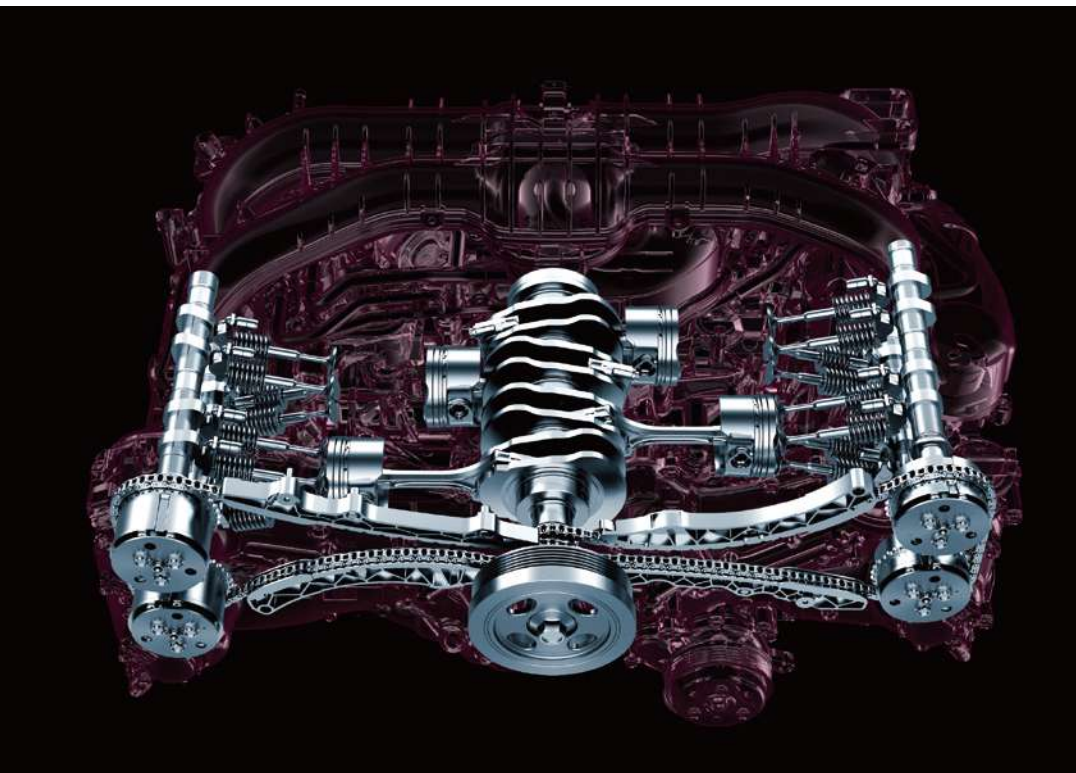
動力性能と環境性能を高次元で両立する2.0ℓ ハイパフォーマンス“DIT”
