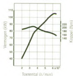
H25A motor vermogenscurve
