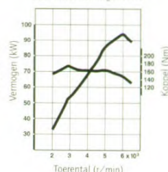
J20A motor vermogenscurve
