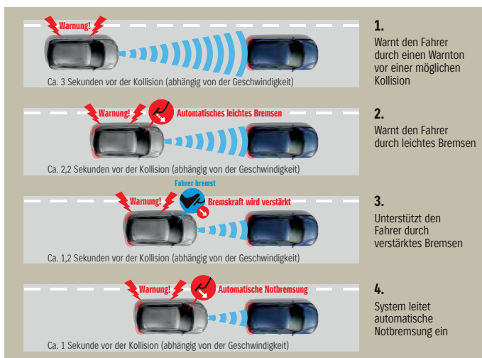
Radargestützte aktive Bremsunterstützung (RBS)
