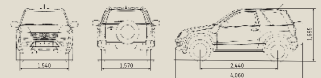
Dimensions - 3 Door
