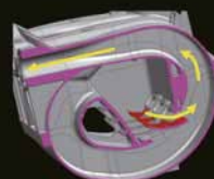
Nouveau collecteur d'admission à longueur variable
