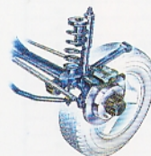
Voorwielophanging met starre as, schroefveren en stabilisatorstang
