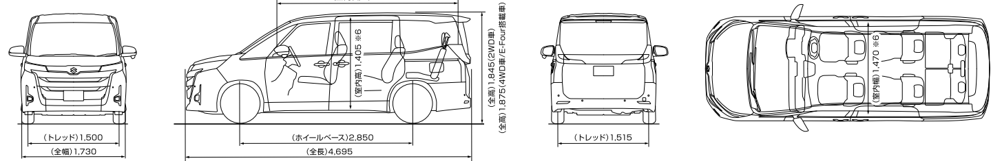
■寸法図 (HYBRID G) 単位:mm
