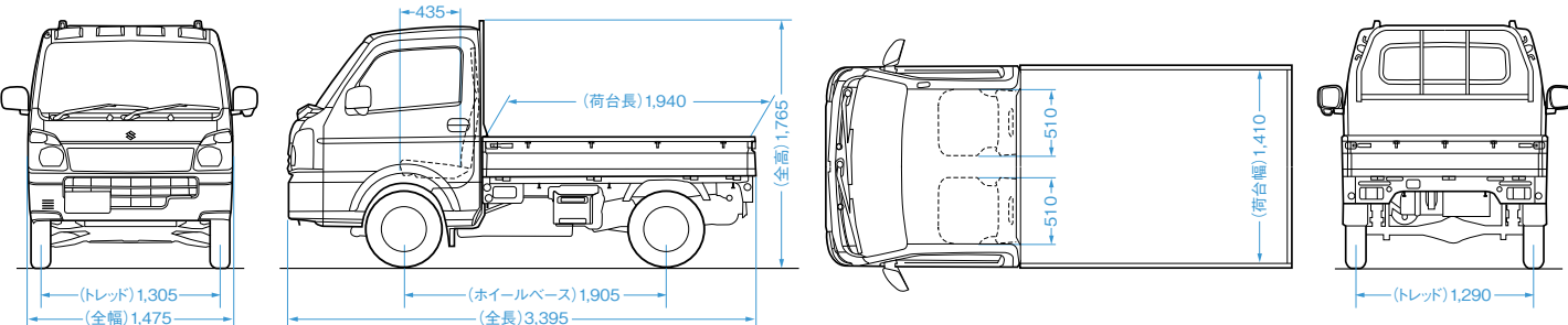
寸法図(KCエアコン・パワステ) 単位:mm
