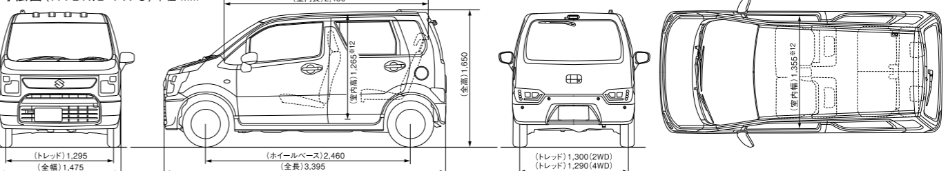
寸法図 (HYBRID FX-S) 単位:mm
