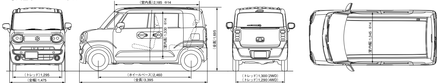
寸法図 (HYBRID X) 単位:mm
