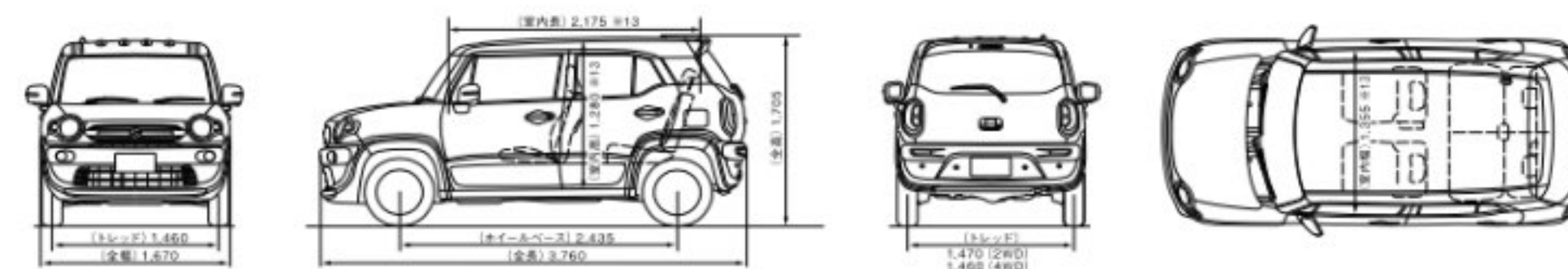
寸法図 (HYBRID MZ) 単位:mm
