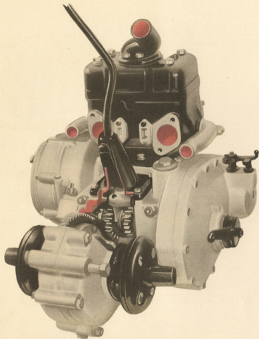
Das gesamte Triebwerk des DKW-Front ist zu einem einzigen völlig geschlossenen Block gefügt.
