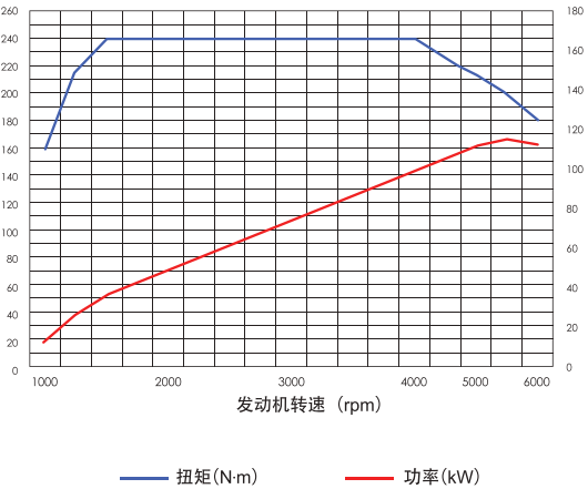
第八代 Ecotec 1.3T SIDI 直喷涡轮增压发动机功率与扭矩图
