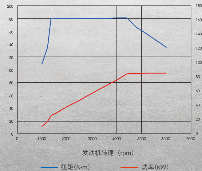
1.0T SIDI 直喷涡轮增压发动机功率与扭矩图
