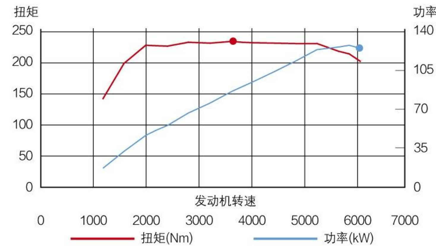
1.6T涡轮增压发动机功率与扭矩图
