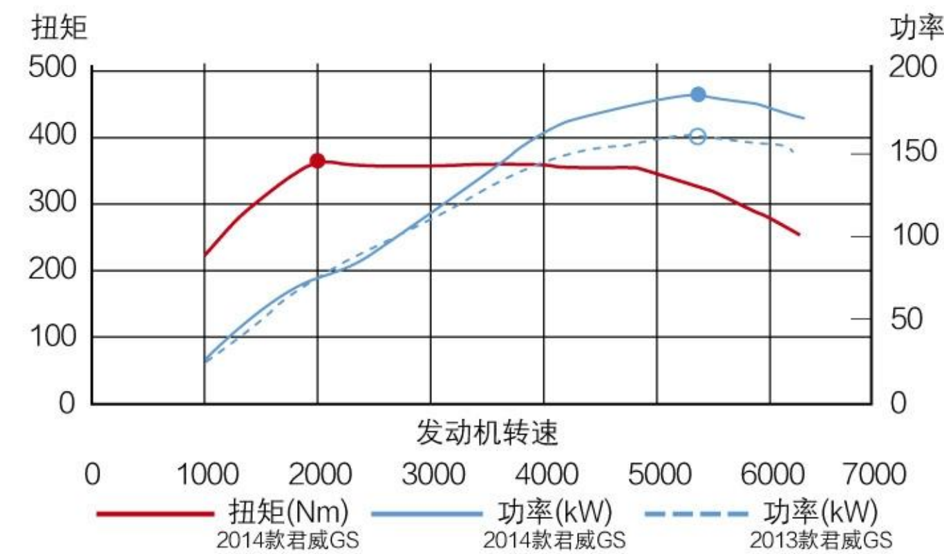
2.0T双涡管直喷增压发动机功率与扭矩图
