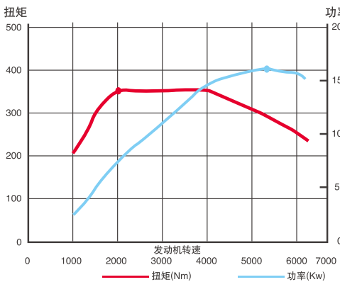
2.0L Turbo DI直喷涡轮增压发动机功率与扭矩图
