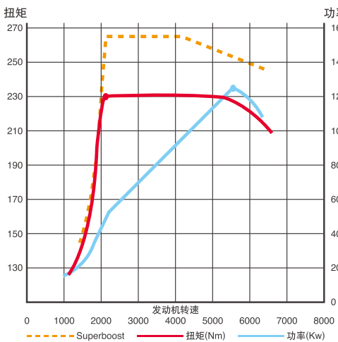
1.6L Turbo涡轮增压发动机功率与扭矩图
