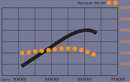
3.8L V6
