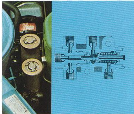
Rembekrachtiging met dubbele remcilinder en veiligheidsklep ter voorkoming van blokkerende achterwielen.
