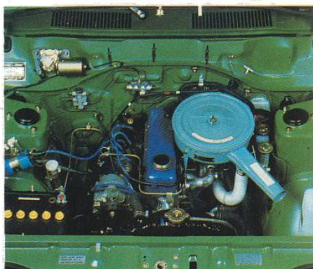
Beroemde 4-cilinder, 1200 cc Nissan motor. In talloze rally's beproefd op betrouwbaarheid en uithoudingsvermogen.
