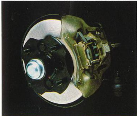
Schijfremmen vóór en trommelremmen achter, met bekrachtiging, om zelfs bij hoge snelheden veilig en op tijd te kunnen remmen.
