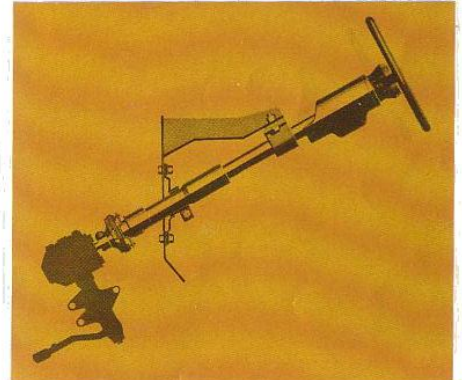
Met het oog op veiligheid ontwikkelde Datsun een samendrukbare stuurinrichting op basis van het stuurkogelkringloop-principe.
