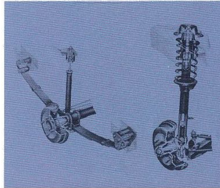
Na landurig testen koos men onafhankelijke voorvering en semi-elliptische telescoopvering achter.
