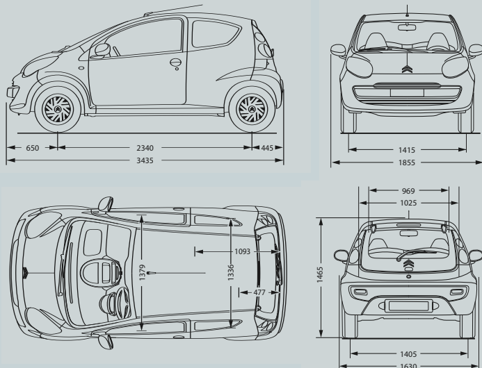
3 Door
