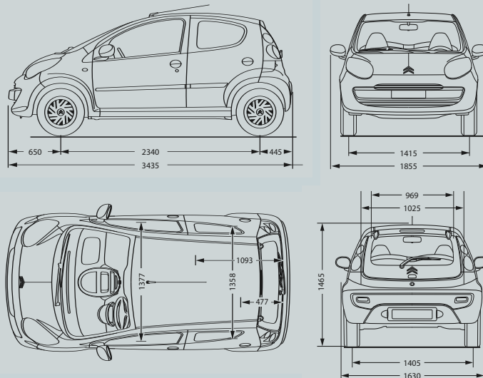
5 Door
