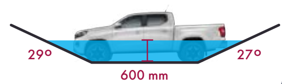
CAPACIDADE DE IMERSÃO ÂNGULOS DE ENTRADA E SAÍDA
