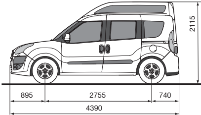
DIMENSIONI TETTO ALTO
