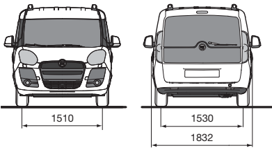
DIMENSIONI TETTO ALTO
