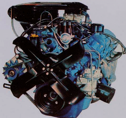
289-cu. in. V-8
