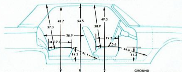
SEDAN DIMENSIONS
