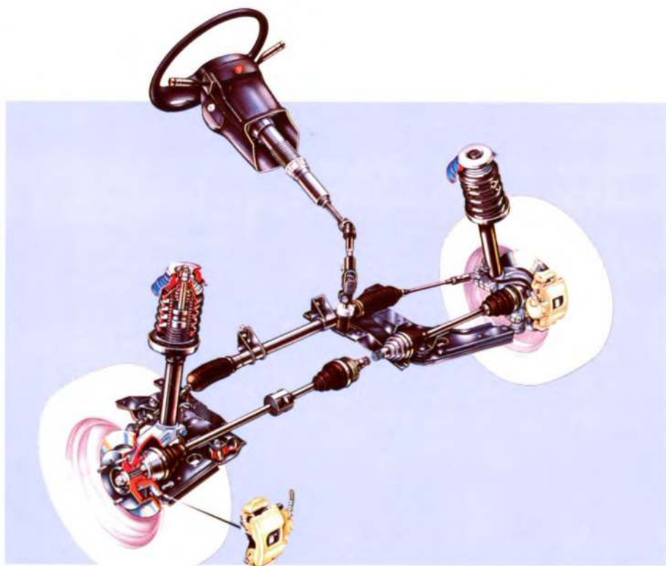
De nieuwe voorwielophanging en stuurinrichting
