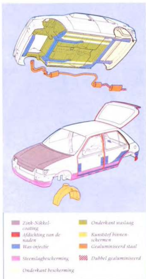
Zó uitgebreid is de behandeling tegen corrosie.
