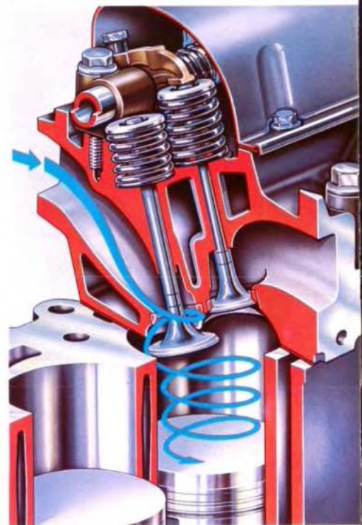
De 1,1 liter HCS-motor met 50 pk/37 kW.
