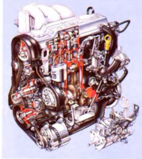
Afbeelding van de opengewerkte 1,8 liter dieselmotor.
