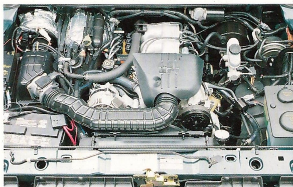
Motor Ford V6 de 4,0 litros, com injeção eletrônica Multi-Port.
