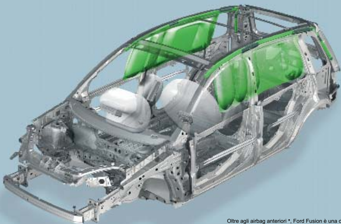
Oltre agli airbag anteriori *, Ford Fusion è una delle prime auto compatte con airbag laterali a tendina.
