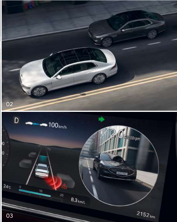
02. 후측방 충돌방지 보조 _ 차로 변경을 위해 방향지시등 스위치를 조작했을 때 후측방 차량과 충돌 위험이 감지되면 경고를 해줍니다. 경고 후에도 충돌 위험이 높아지면 자동으로 차량을 제어하여 충돌 회피를 도와줍니다. 평행 주차 상태에서 전진 출차 중 후측방 차량과의 충돌 위험이 감지되면 자동으로 제동을 도와줍니다.
