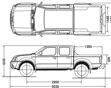
كابينة مزدوجة Double Cab
