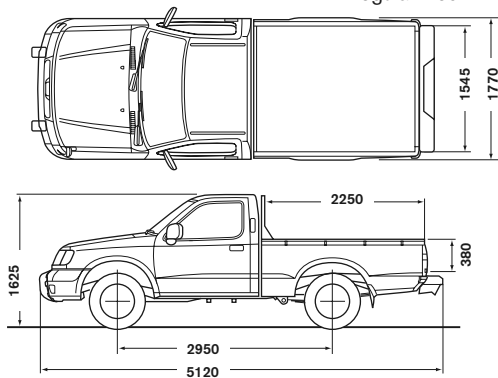
صندوق تحميل عادي Regular Bed
